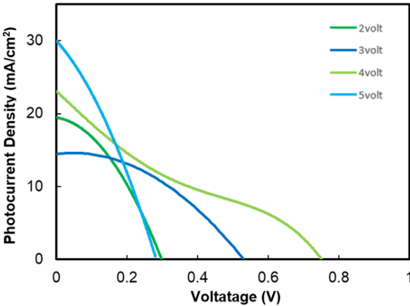
Fig. 9. I-V curves
